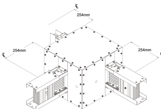
Edgewise Tees
